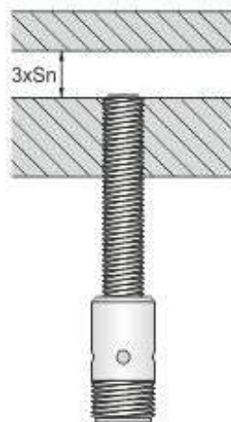
Montaje enrasado
